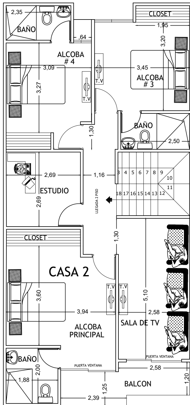
PLANTA ARQUITECTONICA SEGUNDO PISO MEDIANERA
