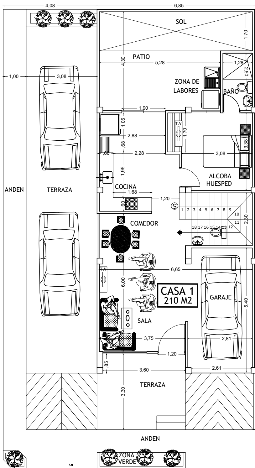
PLANTA ARQUITECTONICA PRIMER PISO ESQUINA
