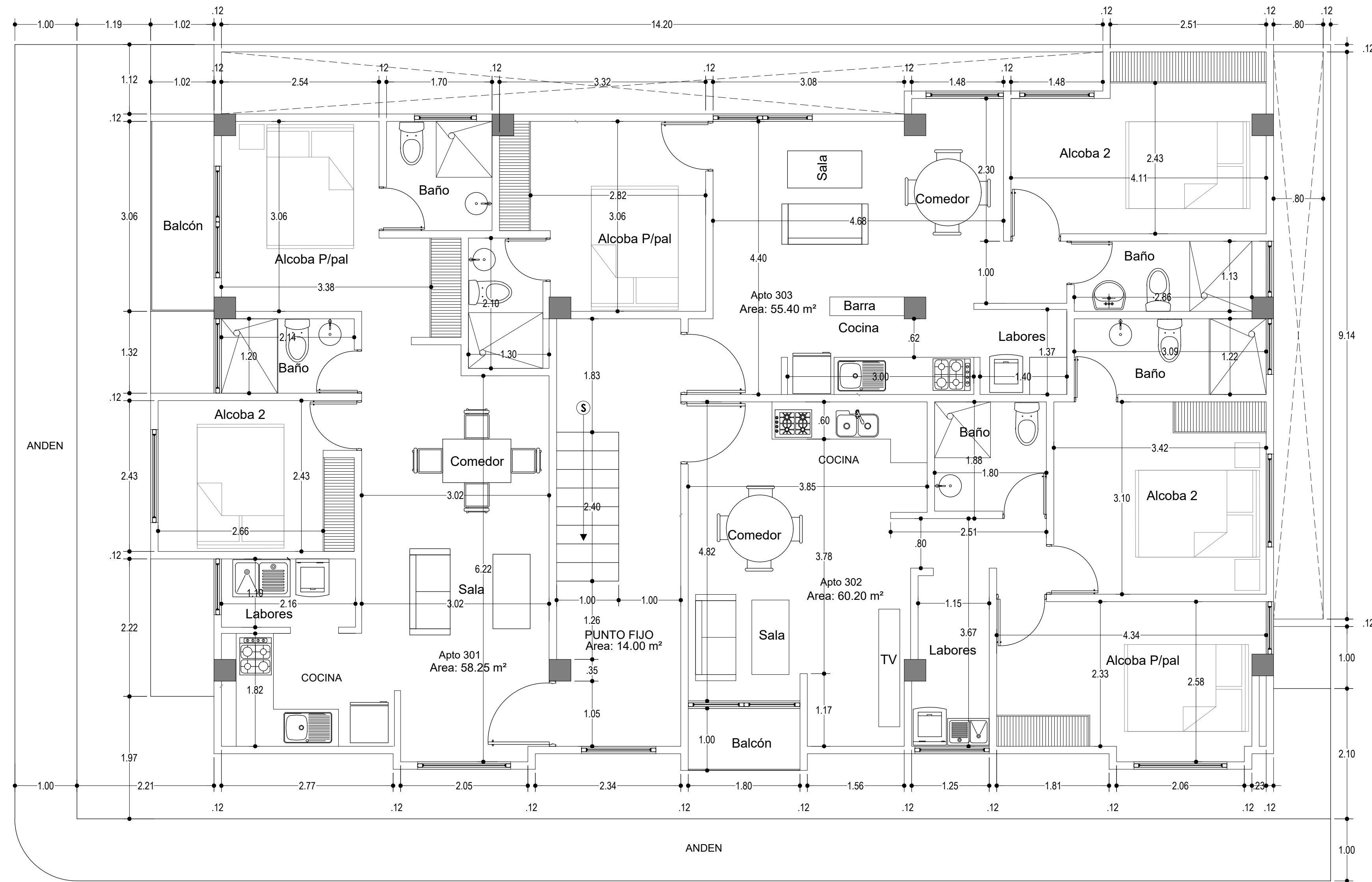
TERCER PISO
