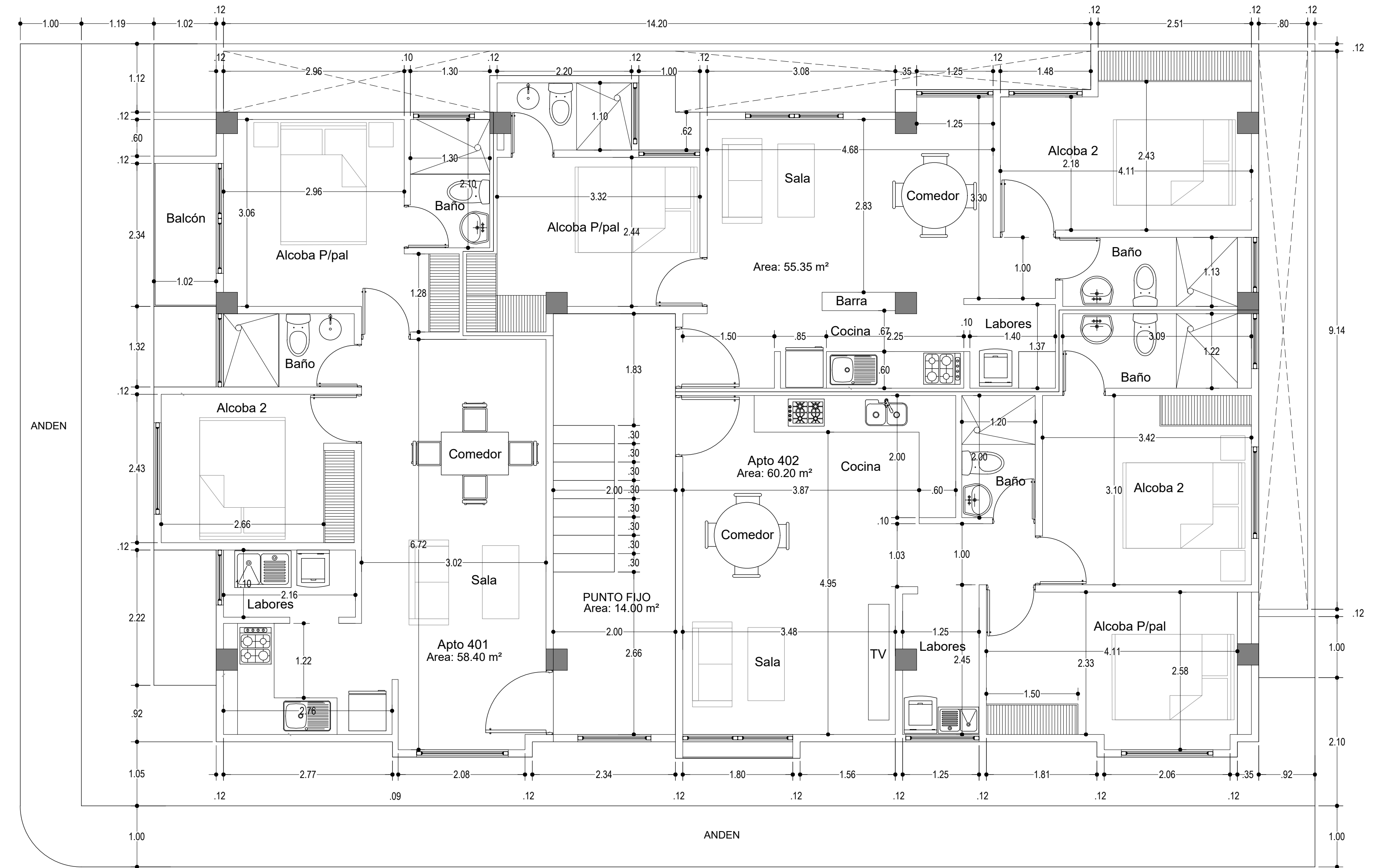
CUARTO PISO
