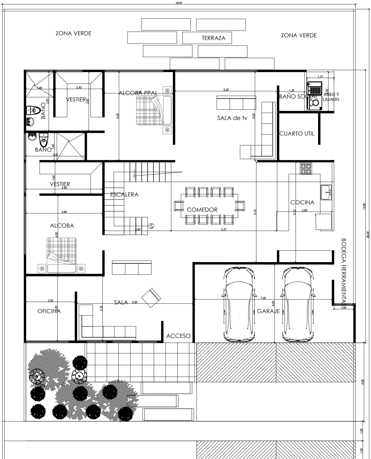
ESCALA 1:50 Planta arquitectónica 1er piso vivienda unifamiliar PROPUESTA 2
